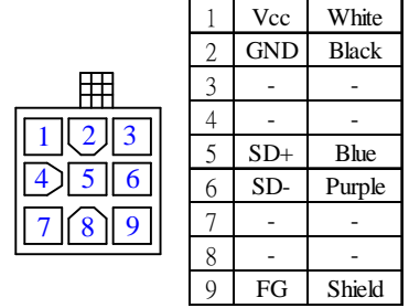
Encoder Wiring
